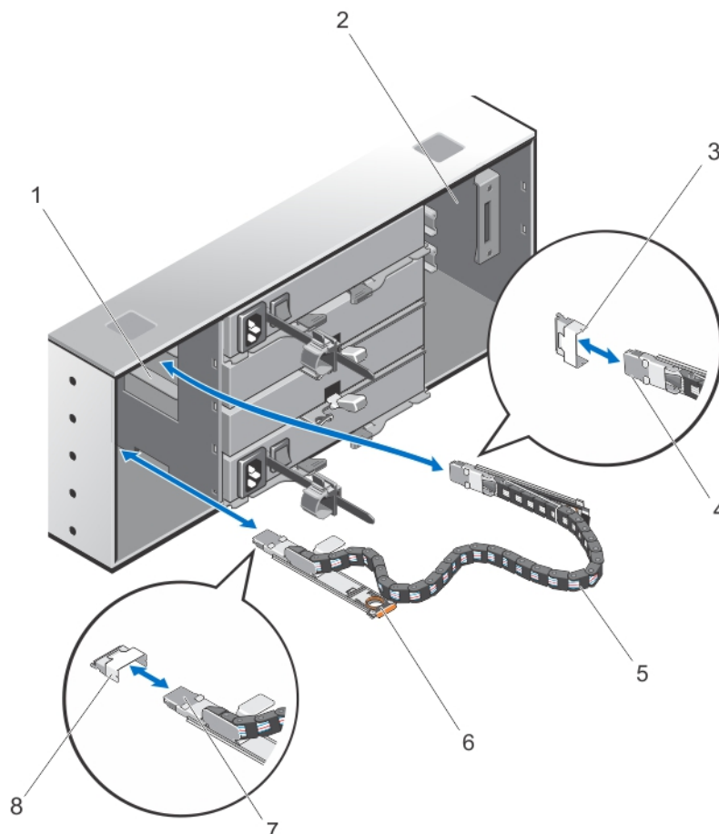
Ilustración 21. Extracción e instalación del cable(s) de cadena SAS
