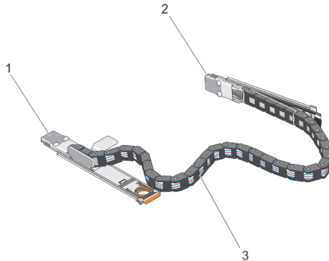
Ilustración 20. Características del cable de cadena SAS
