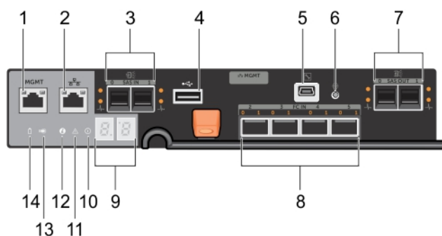
Ilustración 8. Características e indicadores del módulo de la controladora RAID Fibre Channel MD3860f
