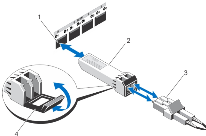
Ilustración 9. Conexión de cable de Fibra óptica
