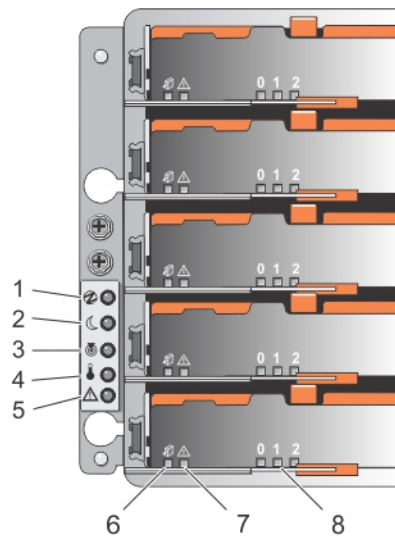
Ilustración 3. Indicadores del panel frontal
