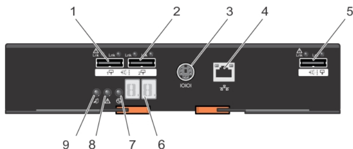
Ilustración 11. Características e indicadores del módulo de expansión MD3060e
