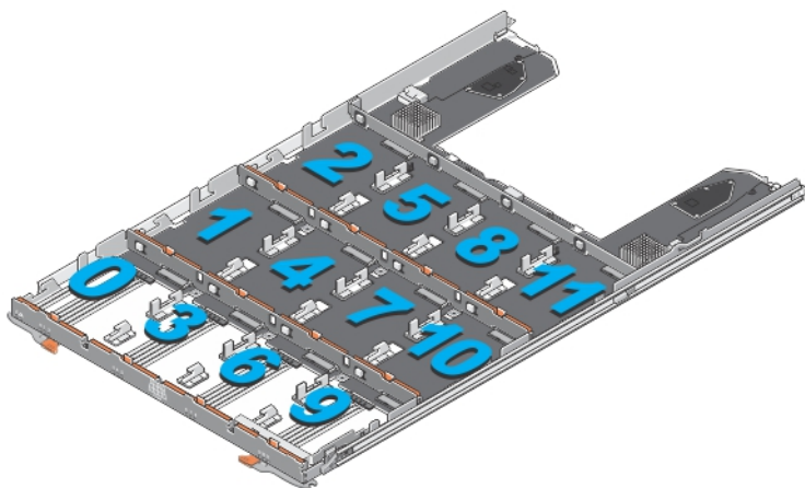
Ilustración 16. Enumeración de la ranura en el cajón del disco
