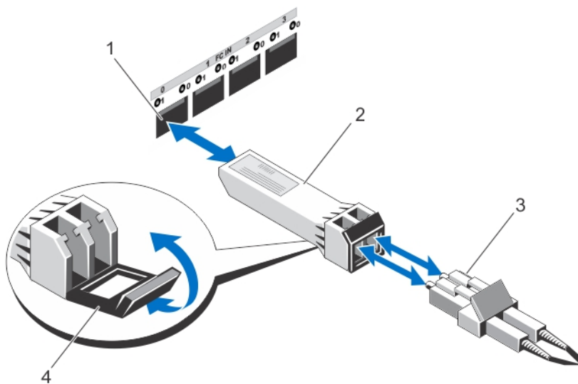
Ilustración 24. Reemplazo del transceptor SFP+
