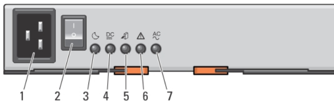
Ilustración 6. Características e indicadores del módulo de suministro de energía
