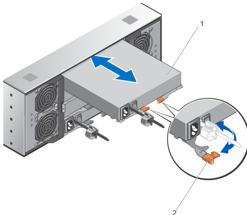
Ilustración 26. Extracción e instalación de un módulo de suministro de energía
