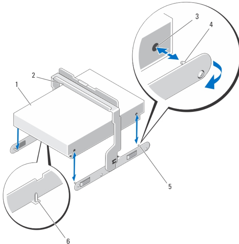
Ilustración 18. Extracción e instalación de un disco físico de 3,5 pulgadas en un portaunidades para discos físicos de 3,5 pulgadas.
