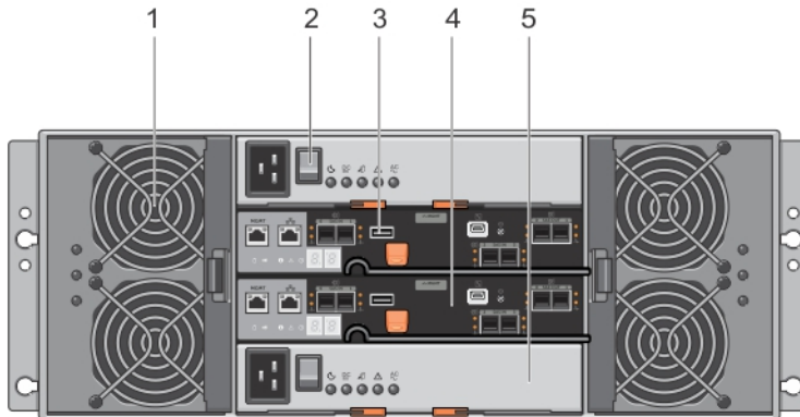
Ilustración 4. Características del panel posterior
