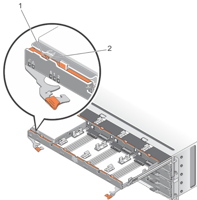
Ilustración 7. Indicadores LED del disco físico
