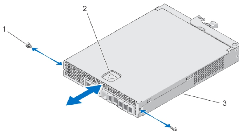
Ilustración 23. Apertura y cierre del módulo de la controladora RAID
