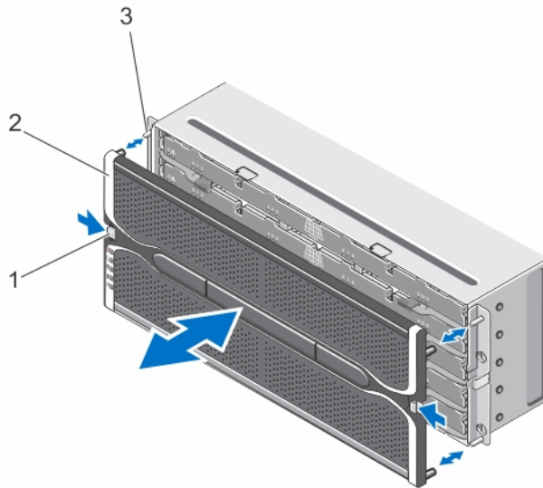
Ilustración 12. Extracción e instalación del bisel frontal
